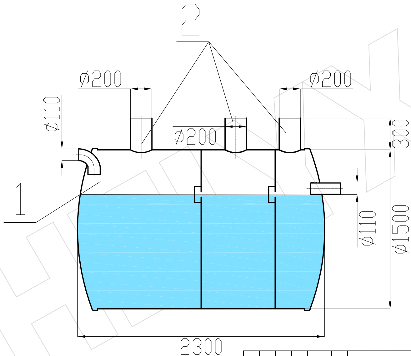
1 Септик V=4000л, D1500, L2300 2 Разгрузочные патрубки
